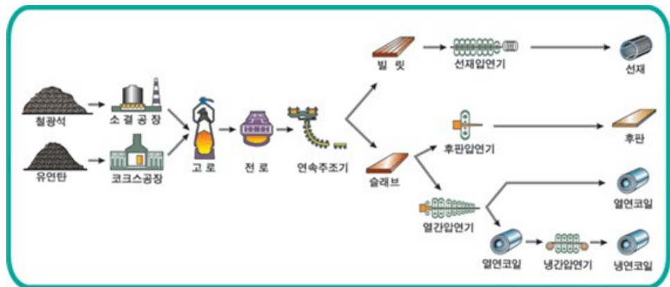
[그림 1] 일관제철과정
