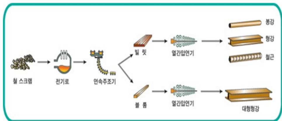
[그림 2] 전기로과정
